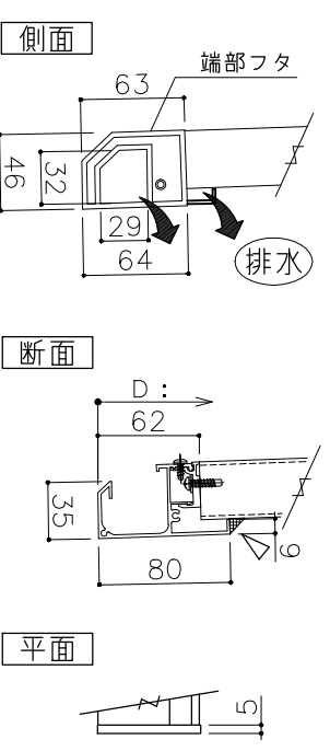
●AD2T (オプション) 先端化粧トイ付
