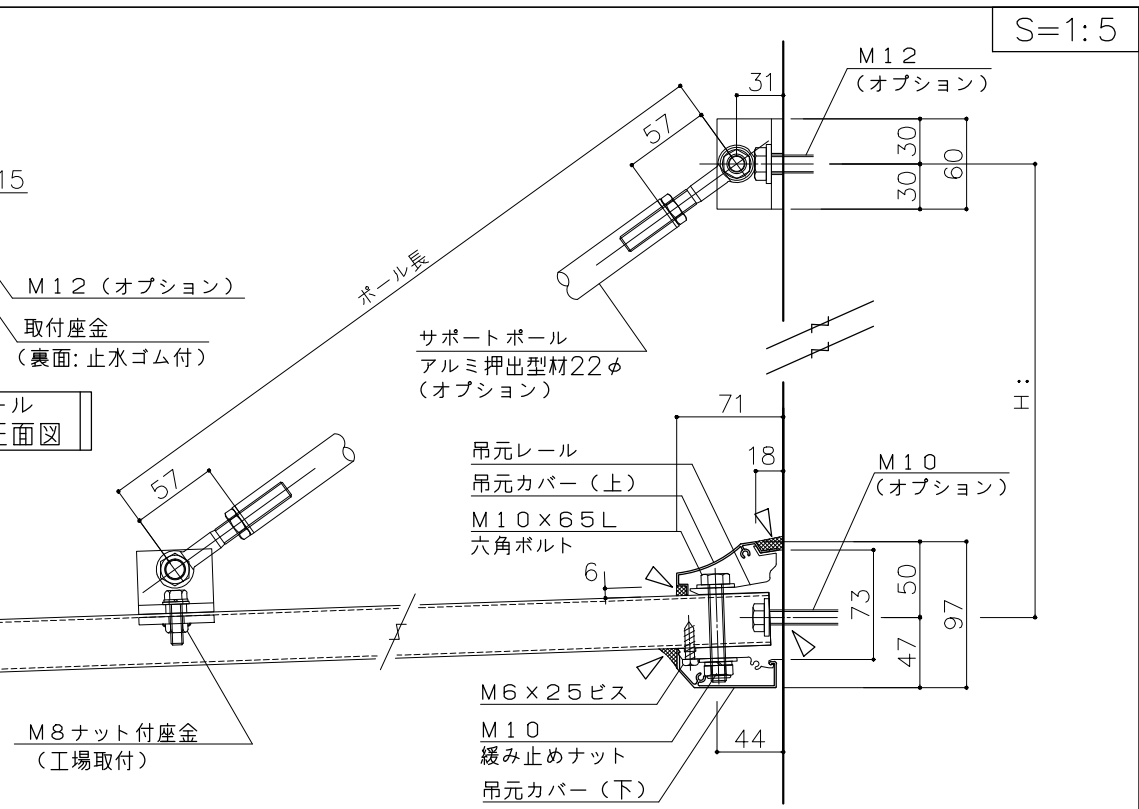
▽: コーキング (別途) 必ず施工してください
