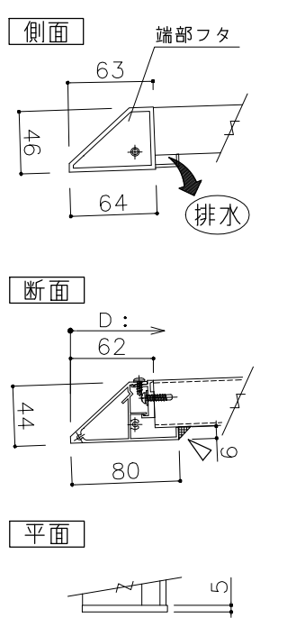
●AD2N (オプション) 先端化粧トイ無
