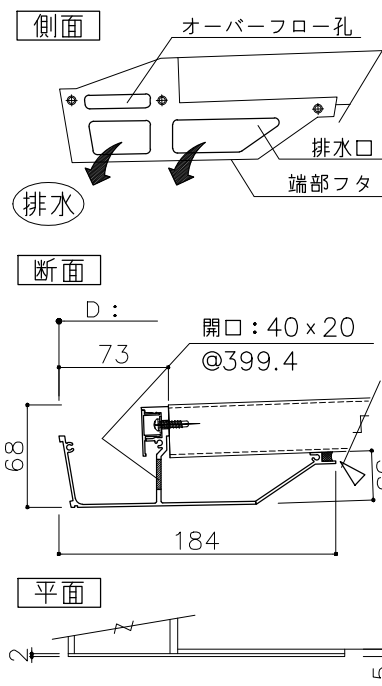
●AD2G (オプション) 先端トイ
