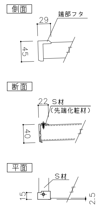
●AD2S (基準) 先端化粧材
