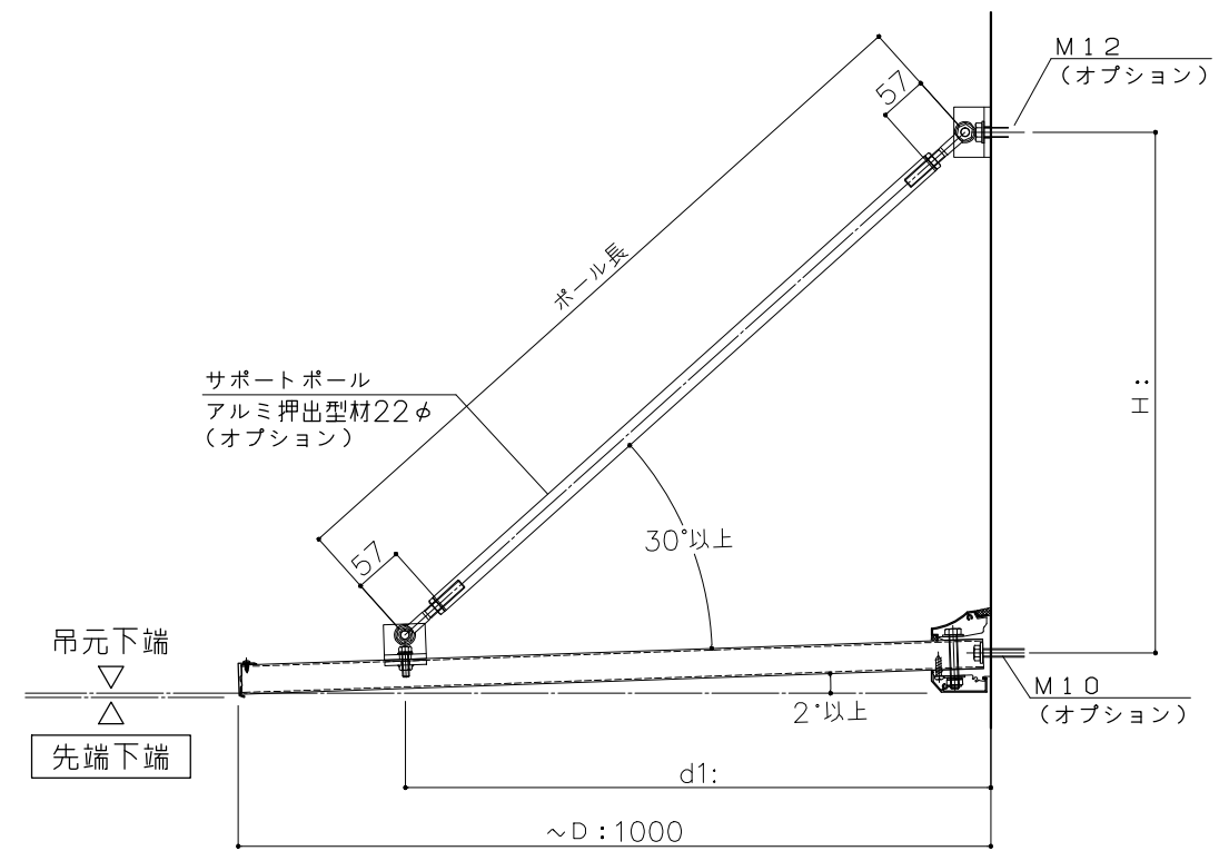
断面図 S=1:10
