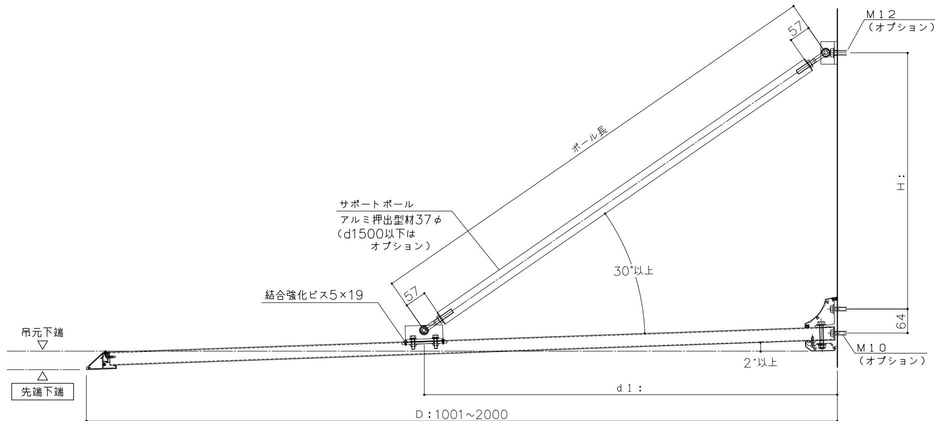
断面图 S=1:10
