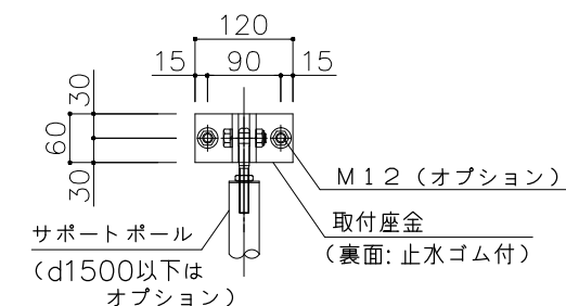
サポートポール 外壁取付き部正面図 S=1:10
