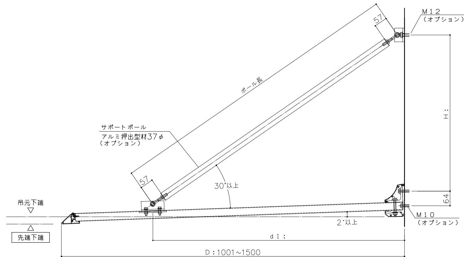
断面图 S=1:10
