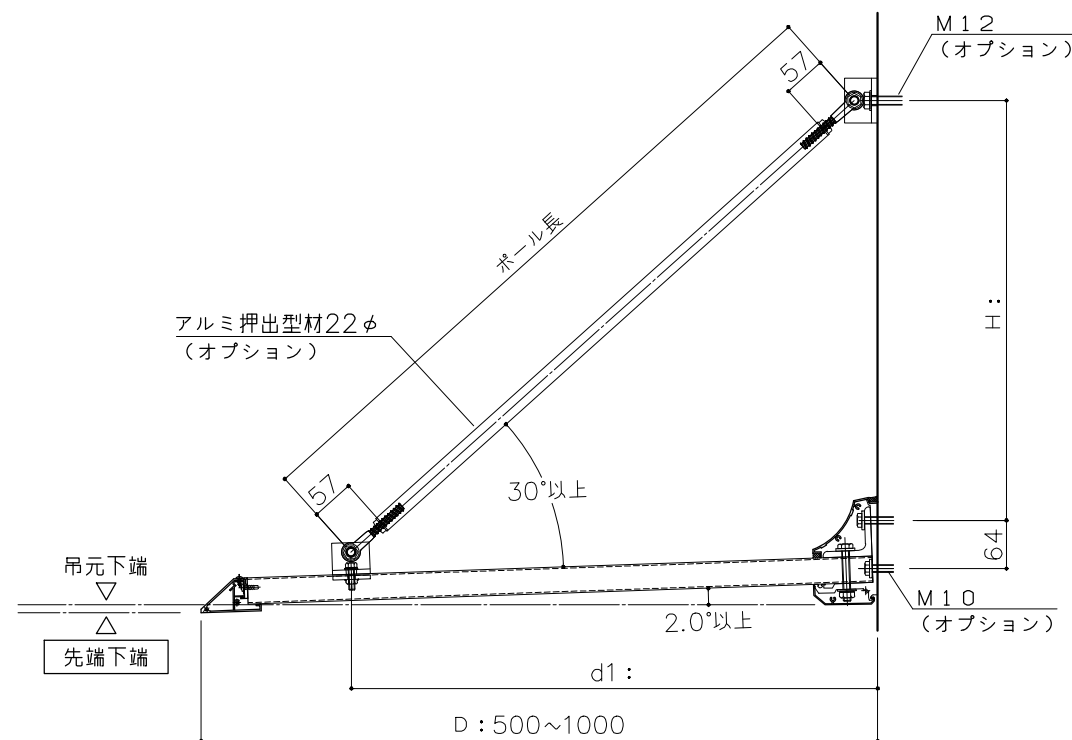
断面図
