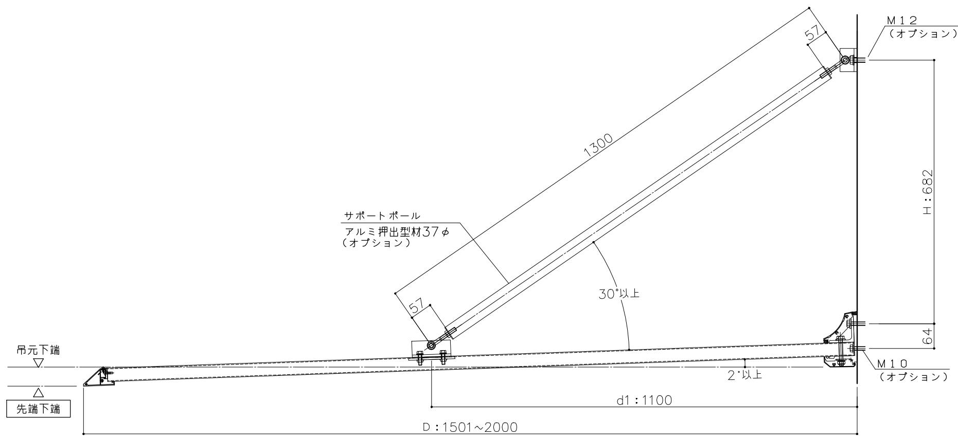
断面図 S=1:10
